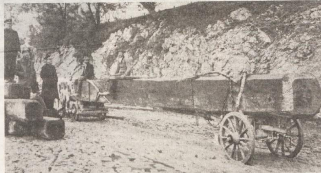
PREVOZ BORDONALA - Bordonala iz Loškega Potoka na železniški postaji na Rakeku. Bordonala je na kvadratičen prerez tesan (ali žagan) tram, dolg 8 do 13 m, debeline od 27 x 27 do 49 x 49 cm. Bordonale so iz naših krajev v prejšnjih časih furali v Trst za ladjedelništvo, po drugih podatkih pa so jih iz Trsta ali z Reke izvažali kot gradbeni material v Francijo.
