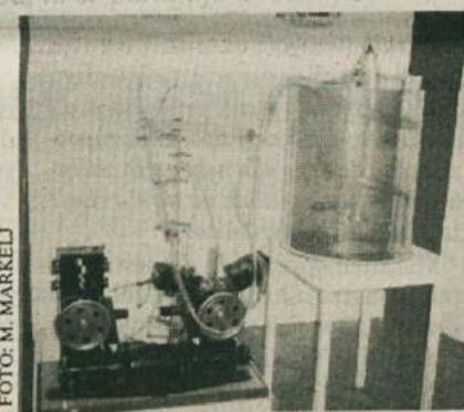
Stroj za zunajtelesni krvni obtok. Izdelala ga je Avtoobnova leta 1958 in z njim je ekipa prof. dr. Mira Košaka opravljala srčne operacije le štiri leta po prvih v svetu.
