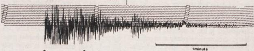
Zapis potresa 11. junija letos, kot so ga zabeležile naprave observatorija Seizmološkega zavoda na Golovcu v Ljubljani.
