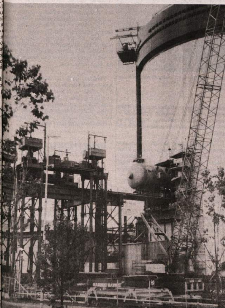
Menjava uparjalnikov ni kdo ve kakšen tehnični problem, so dokazali na Švedskem, kjer so menjavo v svoji jedrski elektrarni Ringhals II opravili lani julija. 300 ton teak uparjalnik, ki je veljal 130 milijonov DEM, so uspeli zmontirati v 72 dne. Na sliki: transport uparjalnika. (Foto: Siemens-Pressbild)
