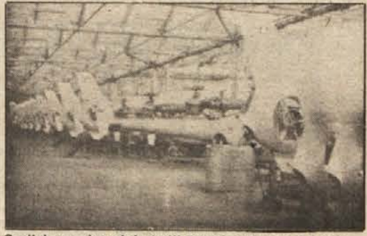
Serijska proizvodnja helikopterjev Gazela SA 341 v tovarni Soko v Mostarju.
