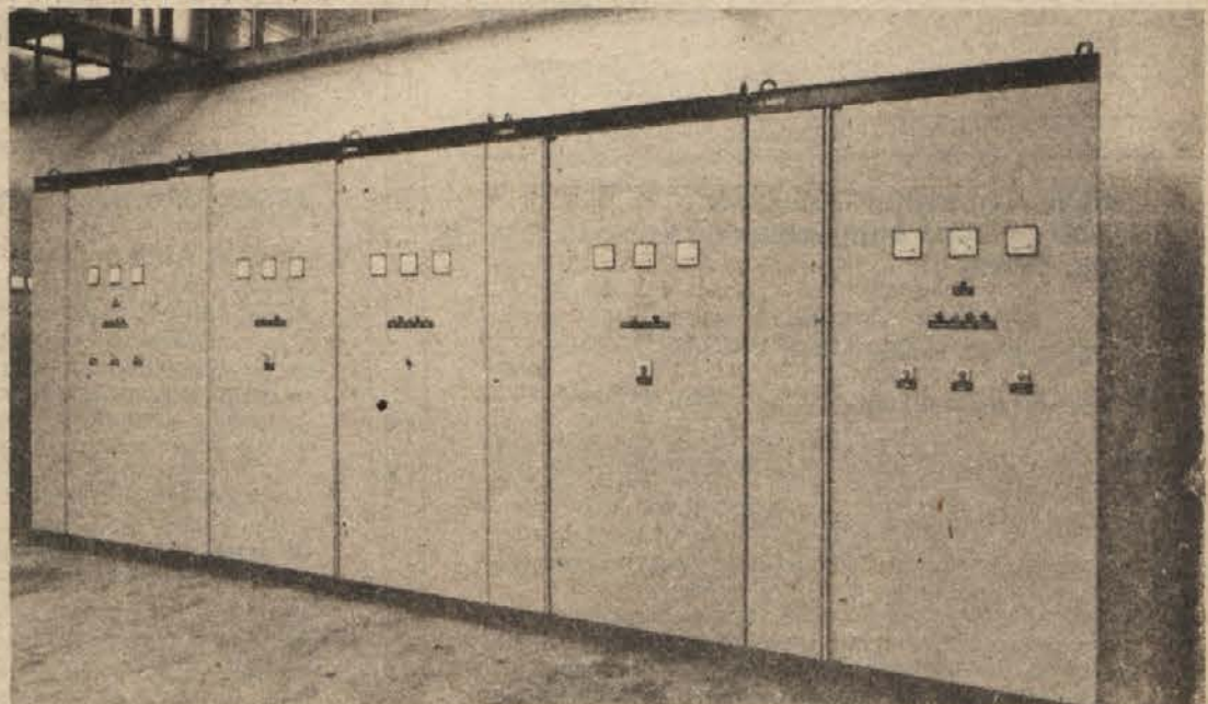
TOVARNA NAPAJALNIH NAPRAV V BRŠLJINU — Brezprekinitveni redundančni sistem izmeničnega napajanja 2x16 KVA za novi telekomunikacijski center v Mariboru.
