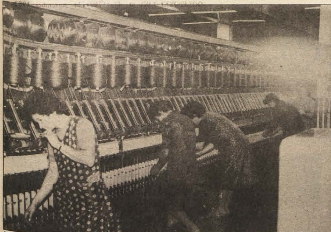
Delavke ob predilnem stroju.
