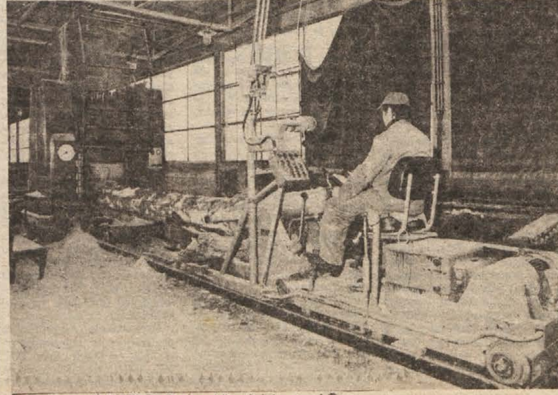
Polnojermernik ETTERER v novi žagalnici - tozd Žaga
