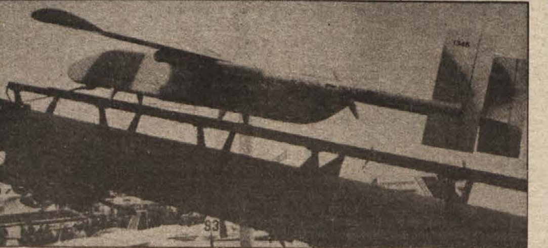
Izraelsko brezpilotno izvidniško letalo je opremljeno s foto in televizijskimi kamerami. V zraku lahko kroži več kot 4 ure s hitrostjo do 100 km na uro, dvigne se lahko na višino 3000 metrov. Letalce lahko ponese 18 kg koristnega tovora. Vsak tak sistem, ki ga sestavlja po šest letal te vrste in ustrezna oprema na tleh, stane približno 2 milijona dolarjev.
