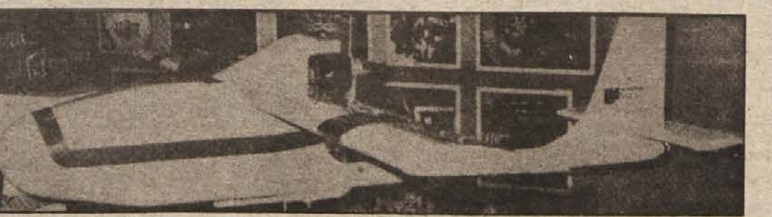
Ameriško miniaturno brezpilotno letalo „E-Systems“ je narejeno iz plastične snovi, namenjeno pa je za izvidovanje in povzročanje elektronskih motenj. Izdeljujejo ga v treh verzijah, ki tehtajo po 9,16 in 41 kg, preletijo pa lahko 335, 390 in 260 kilometrov dolgo pot.
