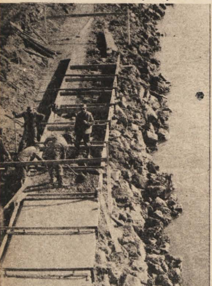
SAVO BODO UKROTILI , da se ne bo več razlivala po poljih. Na sliki je pogled na gradbišče pod starim mestom v Brežicah, kjer bodo dočeli nasip že požira prve kubike betona, gramoz in drugega nasipnega materiala. Z zavarovanjem levega rečnega brega bodo rešili pred poplavami okoli 1000 hektarov plodnih površin. (Foto: Jožica Teppey)
