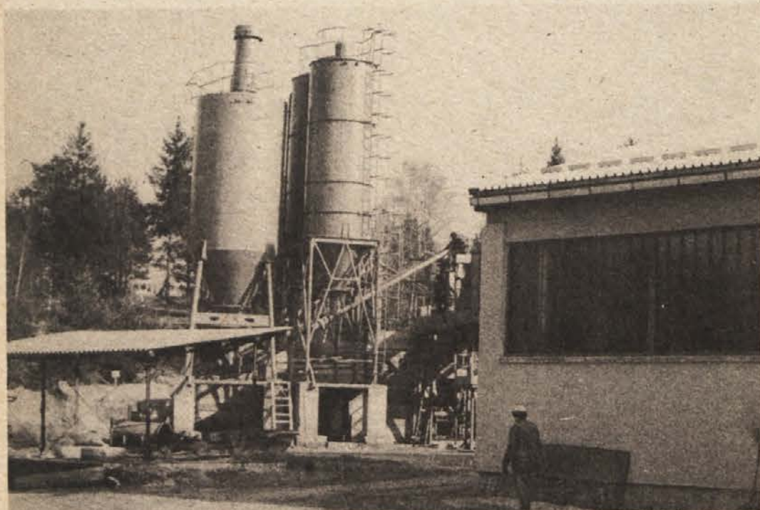
TOZD INDUSTRIJA GRADBENEGA MATERIALA v Kanižarici oskrbuje z gradbenim materialom in izdelki
