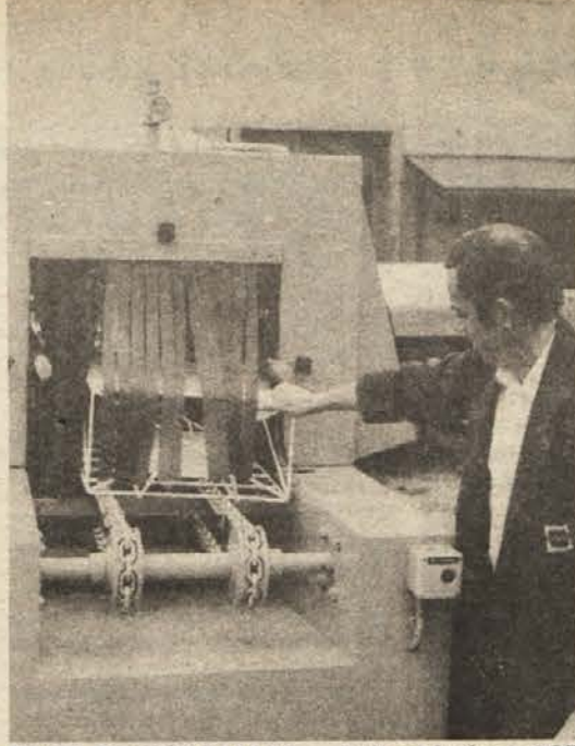
EDINI PROIZVAJALCI – Delavci krškega SOP so ponosni, ker so na nedavnem vinskem sejmu v Ljubljani največ zanimanja poželi prav njihovi stroji za živilsko industrijo. Gre za stroje za prebiranje in pranje sadja in stroje za pranje embalaže (na sliki), ki jih izdelujejo le v Krškem. (Foto: Perc)
