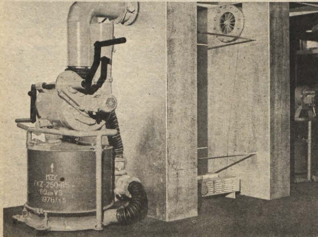
Ventilacijske naprave
