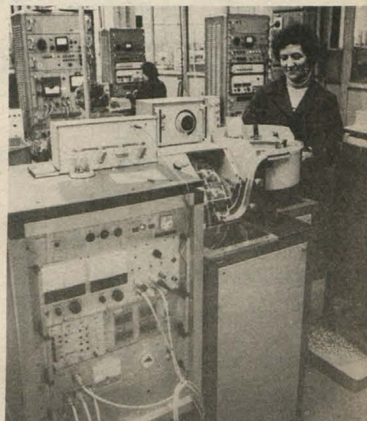
Merilni avtomat MA 10 domače konstrukcije in izdelave
