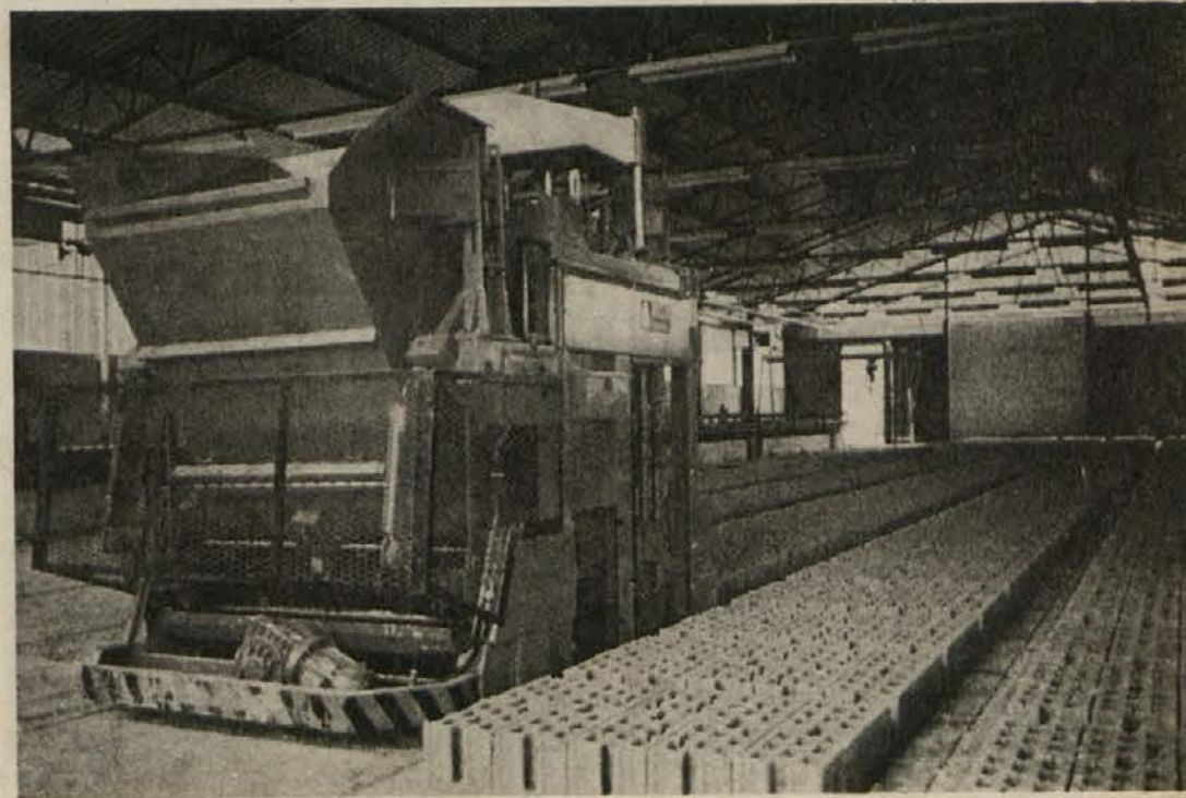
Samohodna vibracijska stiskalnica SVS 1735
