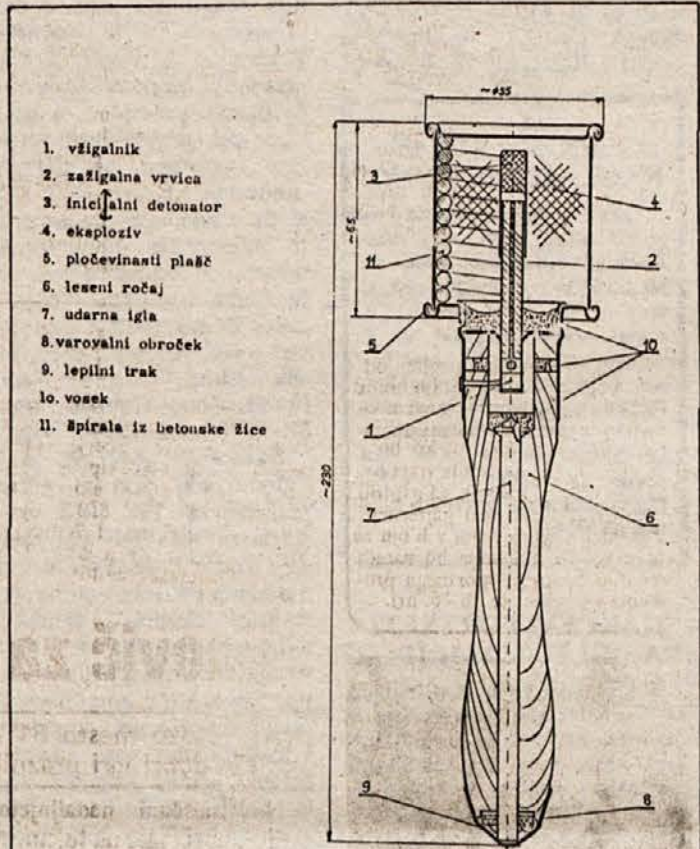
PARTIZANSKA IZNAJDLJIVOST: v orožarski delavnici na Podstenicah izdelana ročna bomba
