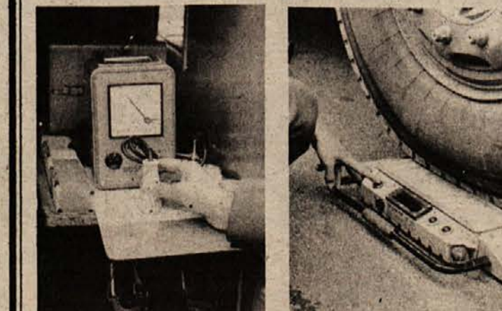
Tudi tokrat je kazalec pokazal preveliko količino strupenih izpušnih plinov.
