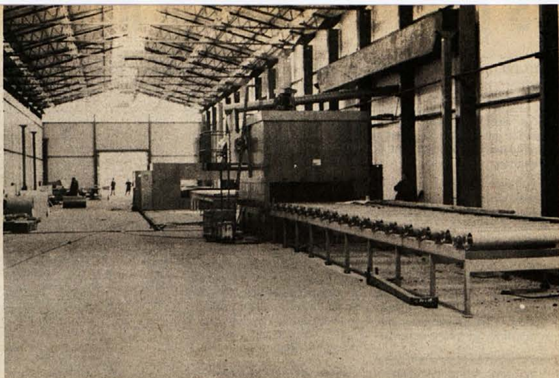
ZA ZAŠČITO JEKLA — Pogled na novo, 90 metrov dolgo linijo za antikorozijsko zaščito jeklenih konstrukcij še ni popoln. Med poročanjem so nanjo montirali še peskalno napravo.
