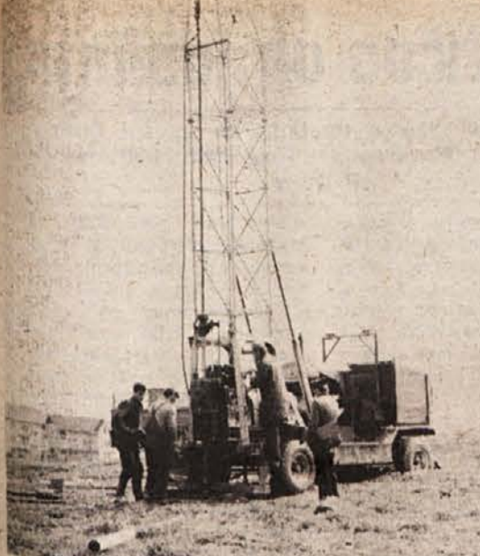
ZA VIADUKT — Delavci ljubljanskega „Viadukta“ so začeli s preiskavami tal na trasi bodočega industrijskega tira za tovarno IMV v Novem mestu. Industrijski tir bo tekkel preko Težkega potoka po viaduktu. Za tovarno je ta prometna povezava življenjsko važna. (Foto: Markelj)
