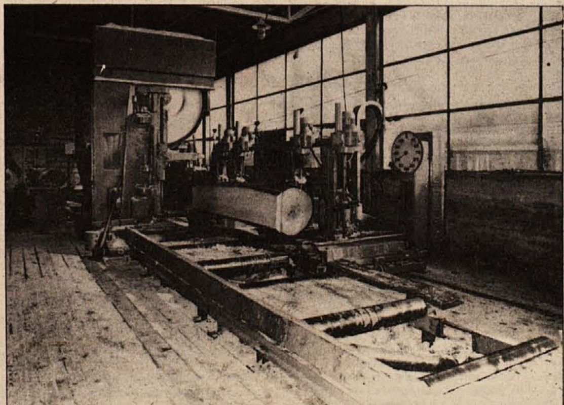
Tračna žaga (brenta) v novi žagalnici TOZD „ŽAGA“
