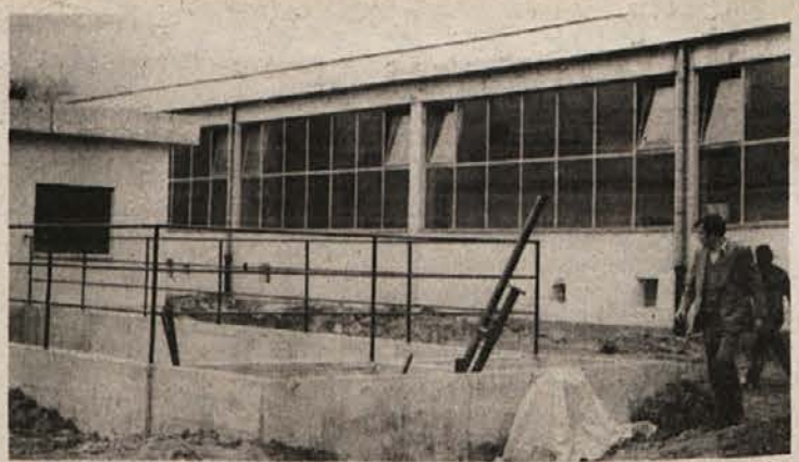
NOVA GALVANIKA — V Inkopu urejajo novo avtomatsko galvansko linijo (v dvorani na fotografiji) in nove čistilne naprave, katerih del je v prednjem delu fotografije. (Foto: Primc)
