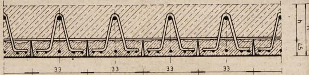
PREČNI PREREZ SKOZI STROP
