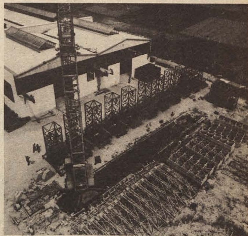
Pogled na montažni prostor in na novo zgrajeni del proizvodne dvorane.
