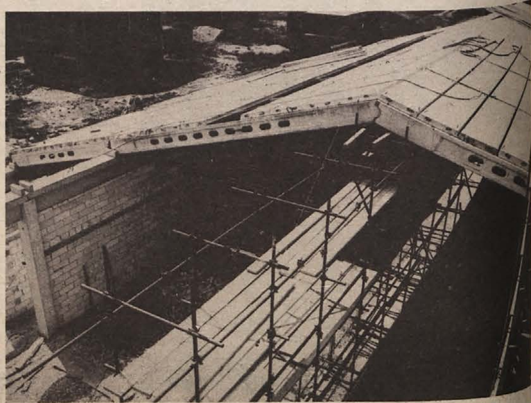
GRADNJA MONTAŽNE HALE „TOGREL“ S STREHO NOVEGA TIPA — DVOKAPNICO — V VELIKI GORICI PRI ZAGREBU
