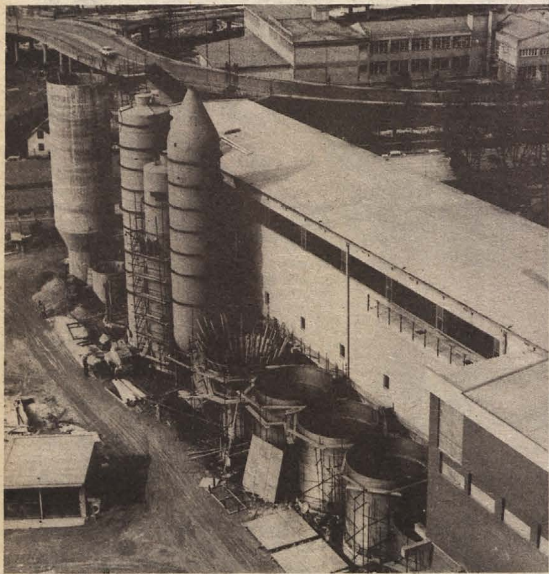
Med največje objekte, ki smo jih zgradili, uvrščamo nedvomno izgradnjo magnefitne celuloze v tovarni „Djuro Salaj“ v Krškem.
