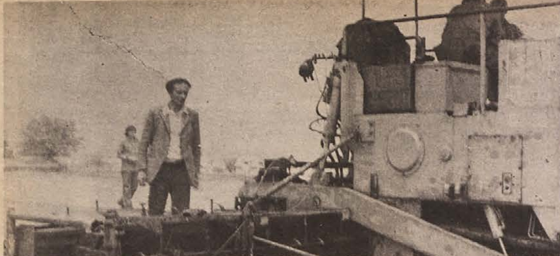
OBVOZNICA V BREŽICAH: Delavci podjetja Slovenija ceste so minuli teden dokončali obvozno cesto, ki so jo speljali od bizeljskega križišča do priključka v tovarno IMV. Delali so z naj sodobnejšimi stroji. Na sliki vidite orjaški finiše, ki lahko asfaltira 16 metrov široko cestišče. Za njim je utrjeval asfalt devetnajststonski valjar, zbitost asfalta pa so merili z izotopsko sondo. (Foto: Jožica Teppey)
