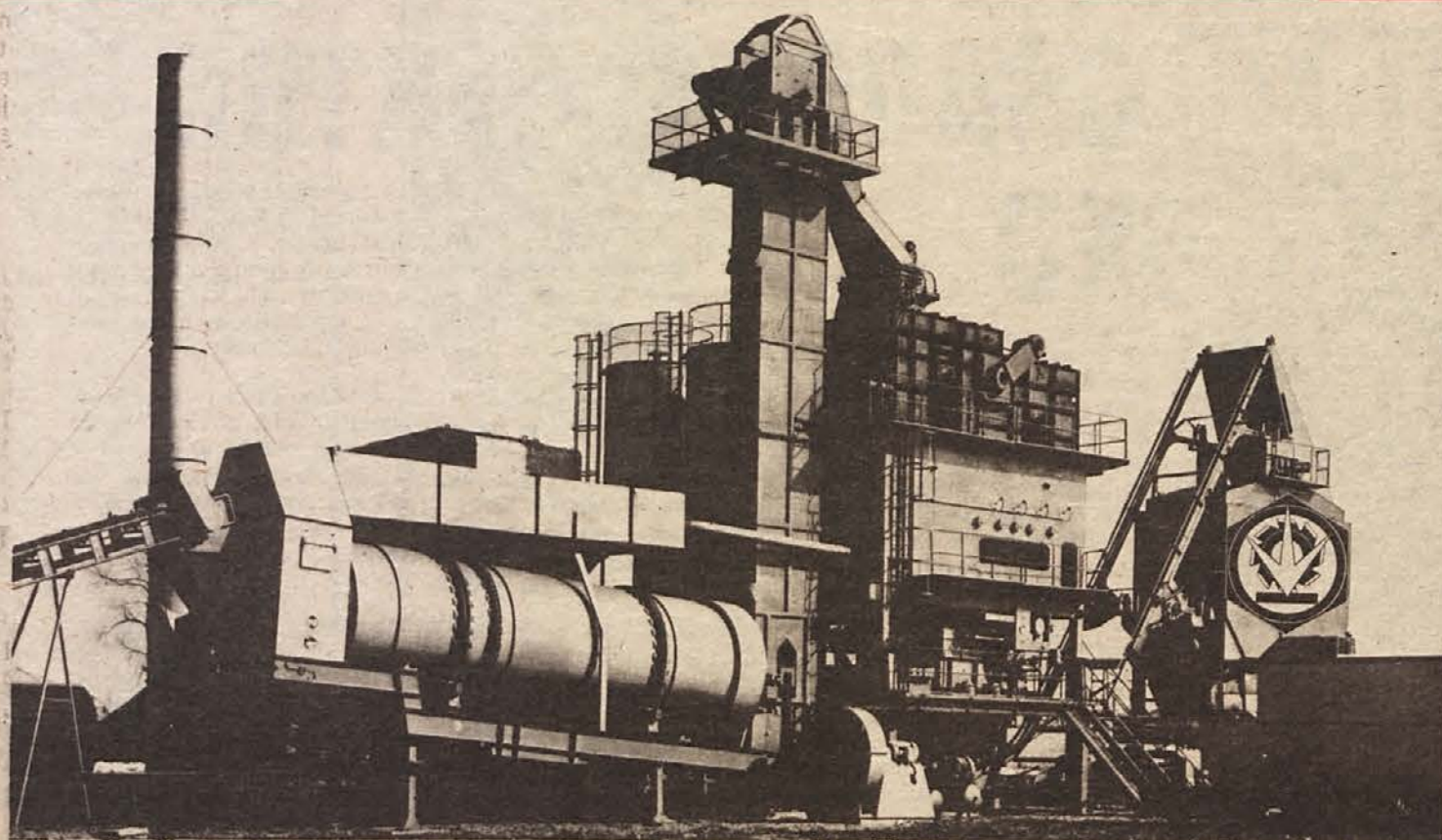
ASFALTNE BAZE so eden najvažnejših proizvodnih programov Kovinarske. Izdeluje jo jih v sodelovanju s firmo Wibau iz ZR Nemčije. Baze imajo proizvodno zmogljivost tudi do 160 ton asfaltne mešanice na uro. Z njimi so predvsem uspeli na domačem trgu, prodrli pa so tudi na tuja tržišča. Doslej so jih izvažali v Čehoslovaško in v Alžir, dogovarjajo pa se tudi o dobavi asfaltnih baz v Sovjetsko Zvezo, Madžarsko, Romunijo, v arabske dežele in celo na Kubo.
