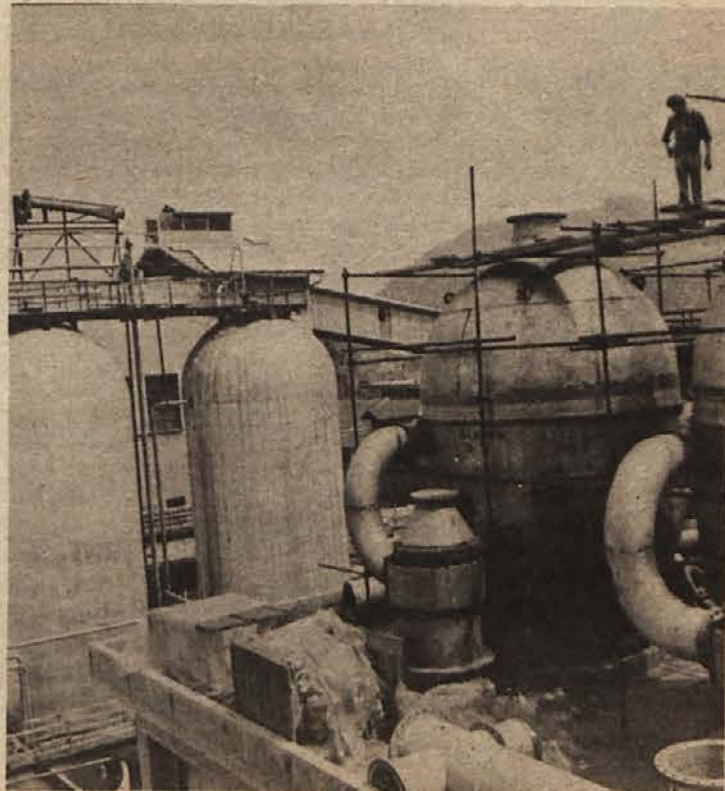
Objekt: UPARILNICA — izdelan v Kovinarski, med montažo v tovarni „Djuro Salaj“.
