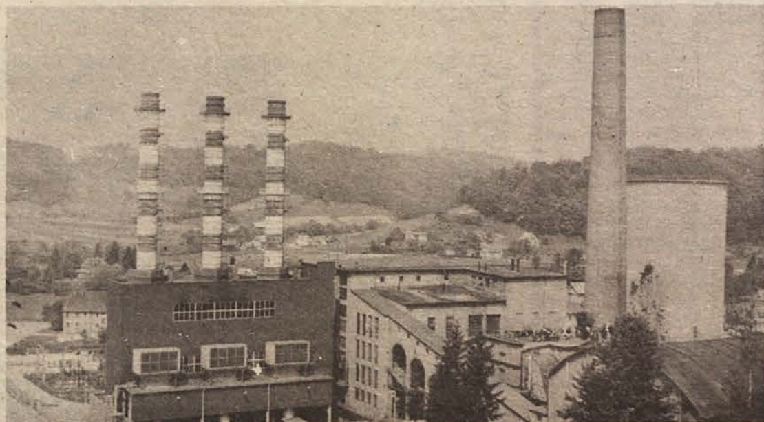
NOVA PLINSKO-PARNA ELEKTRARNA v Brestanici z zračnimi filtri in komandnimi prostori treh plinskih blokov. Na desni je viden del stare termoelektrarne in v ozadju stolp za hlajenje vode.
