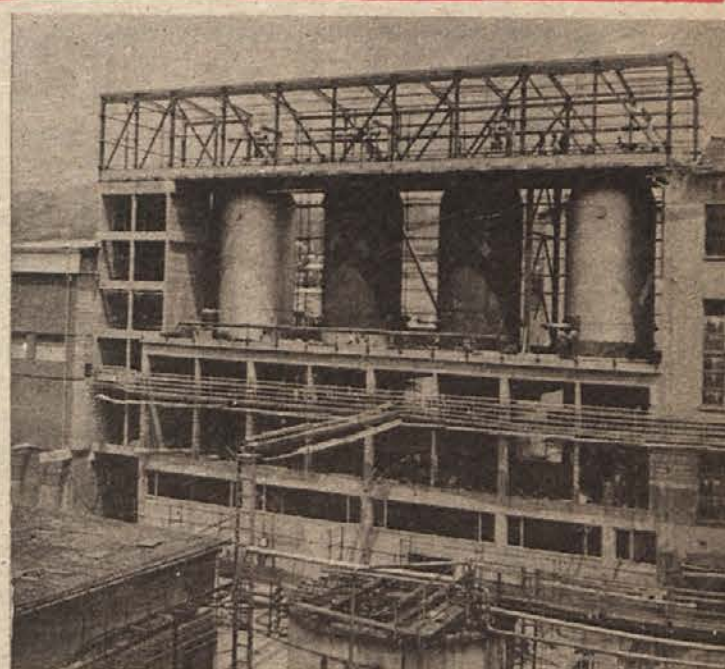
Izredno zahteven objekt, ki so ga naredili za Tovarno celuloze in papirja „Djuro Salaj“ iz Krškega, so kuhalniki. Na sliki: objekt med montažo.
