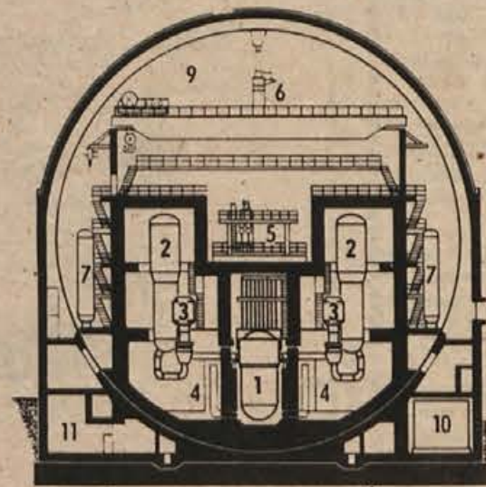
1. reaktorska tlačna posoda in pogoni regulacijskih palic - 2. uparjalnik - 3. črpalka za hladilni medij - 4. betonska ohišja reaktorja, uparjalnikov in črpalik - 5. polinilni stroj - 6. krožno dvigalo - 7. tlačna napajalna posoda - 8. rzušnjača betonska ohišja - 9. varnostna jeklena posoda - 10. posoda za borirano vodo - 11. skladišče za radioaktivne odpadke
