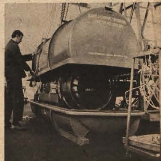
Ko je motor obnoven in pregledan, ga odpremijo v enoto v kovinskem sodu pod pritiskom
