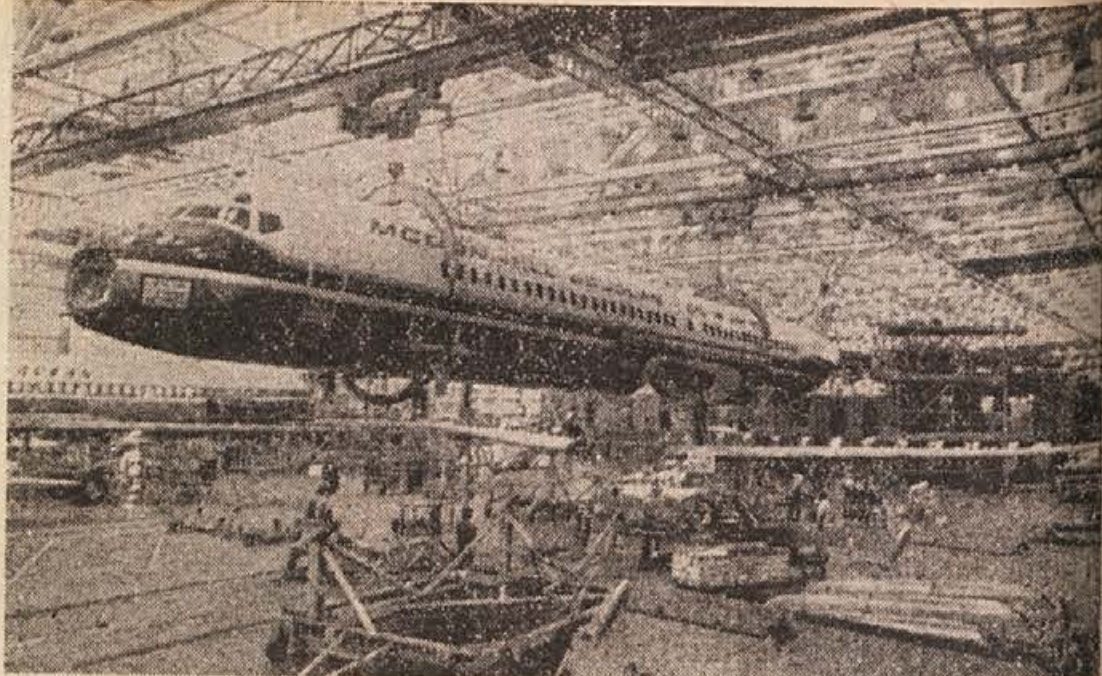
LONG BEACH, Kalifornija - V tukajšnji letalski tovarni družbe Douglas so začeli izdelovati novo izvedenko znanega (in tudi v Jugoslaviji uveljavljenega) letala DC-9. Sedanji tip ima 139 sedežev in je štiri metre daljši od prejšnjega. Menda se za nakup novega modela zanimata tudi dve letalski družbi iz Jugoslavije. Na sliki: pogled v dvorano tovarne, kjer sestavljajo nova letala. (Telefoto: UPI)
