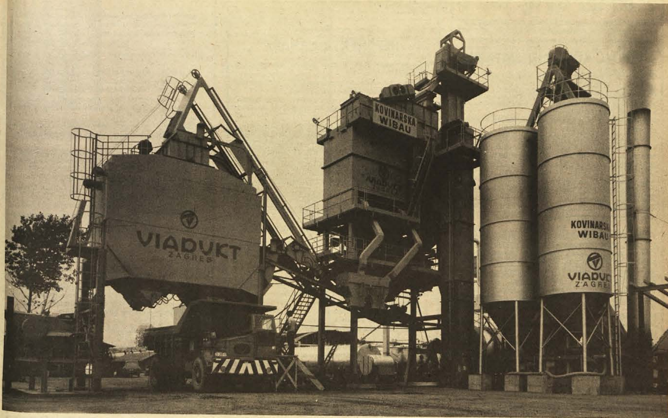
Izdelek Kovinarske iz Krškega. Naprava za izdelovanje asfaltnih mešanic z zmogljivostjo 140 ton na uro.
