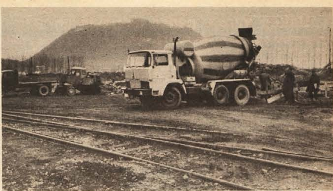
V tovarni papirja v Krškem so zasadili lopate. Do konca zime morajo dokončati temelje in postaviti dvorano za nov papirni stroj. Obratovati bo začel spomladi. Z njim se bo proizvodnja papirja podvojila. (Foto: Zalokar)
