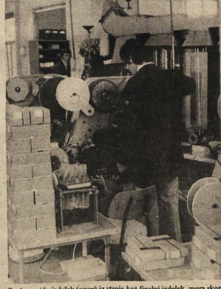
Preden pride izdelek (upor) iz stroja kot finalni izdelek, mora skozi vrsto zapletenih procesov. Enega teh kaže tudi posnetek.
