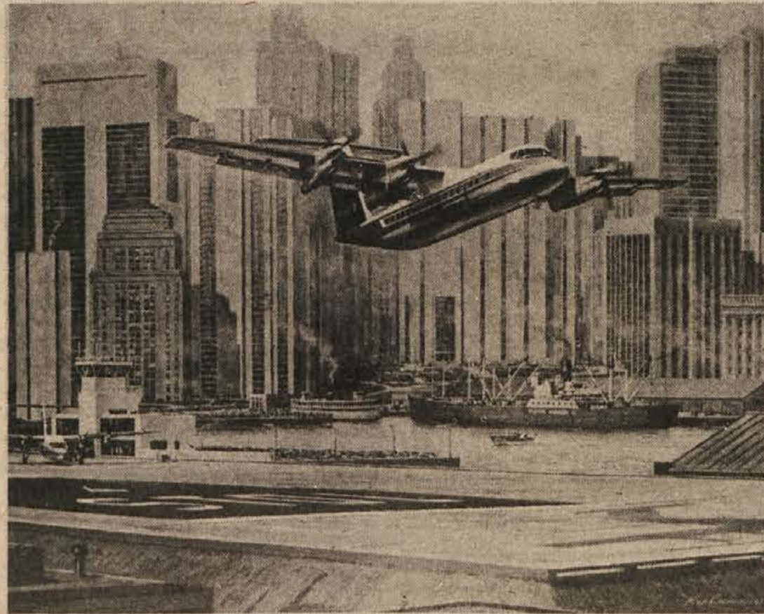
Na sliki je letalo STOL, 48-sedežni kanadski De Havilland DHC-7, s štirimi Pratt in Whitneyevimi turbo-propelerskimi motorji, ko vzleta na 700 metrov dolgi ploščadi tako rekoč sredi mesta
