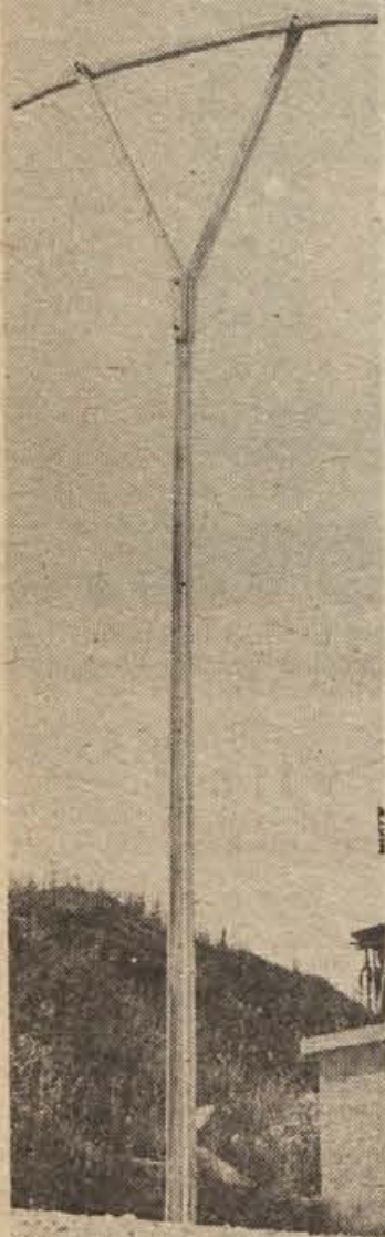
Drog iz prednapetega betona za visokonapetostno omrežje
