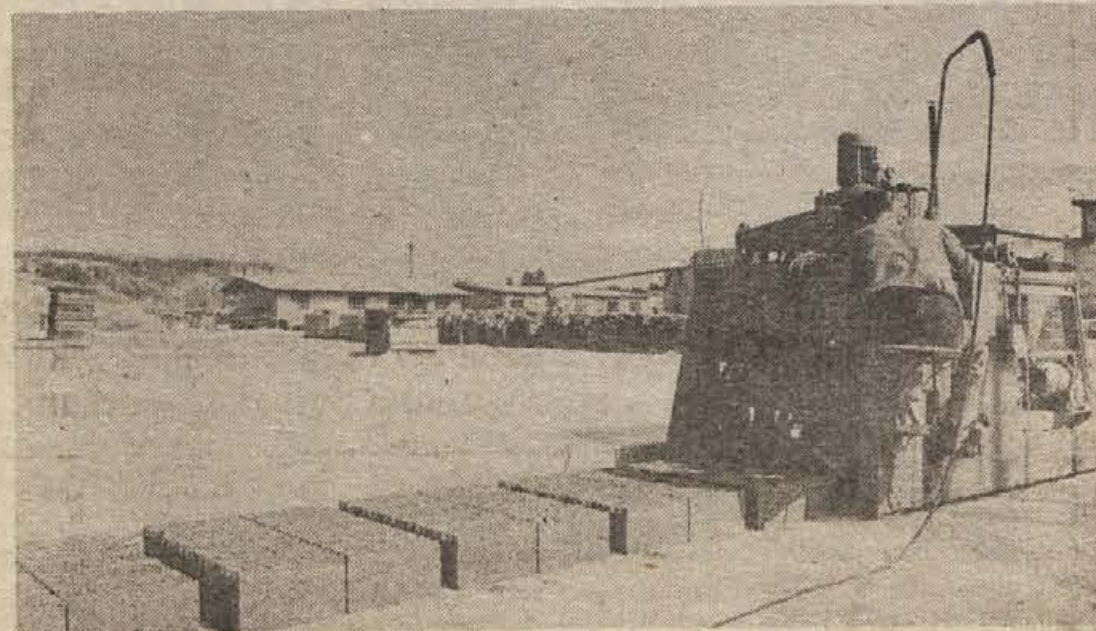
Moderen stroj za izdelavo betonskih votlakov odlaga izdelke na veliki ploščadi v gramoznici na Drnovem
