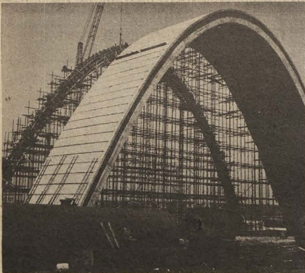
Gradbišče Tovarne dušičnih gnojil v Obiliću pri Prištini
