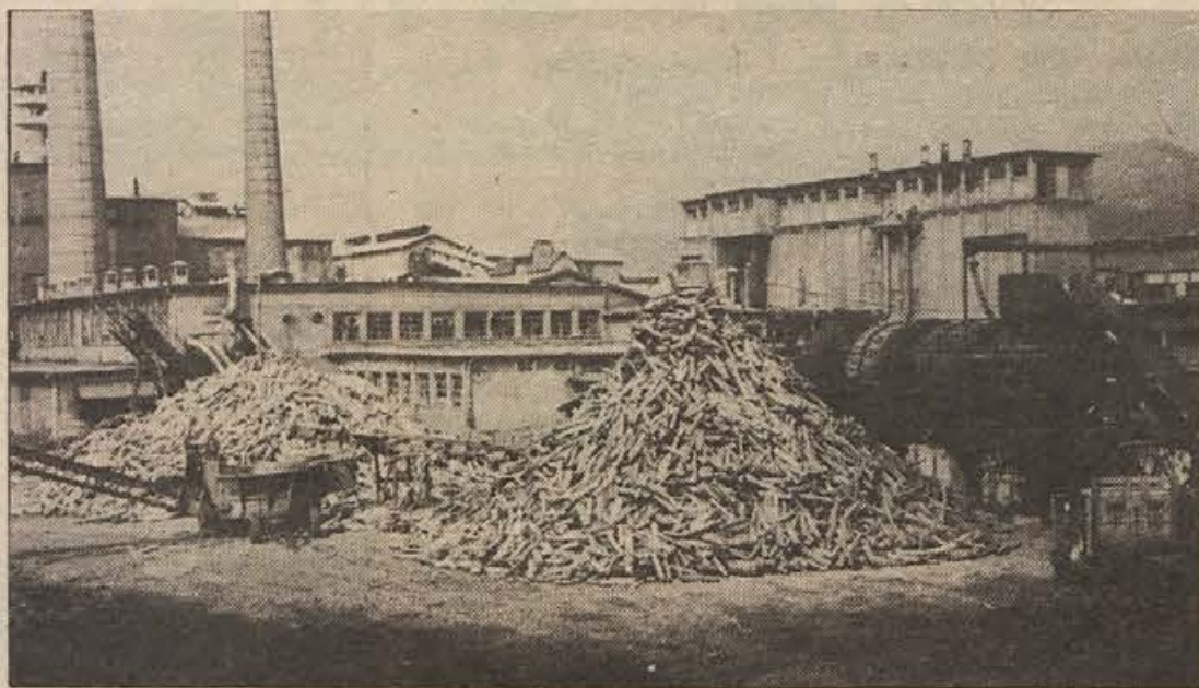
„VELIKA NAPRAVA — Stroj za čiščenje lesa v krški tovarni Celuloze je začela obratovati. Ko bodo dokončani vsi transportni elementi, bo njena zmogljivost preko 1000 prostorninskih metrov lesa na dan. Enako delo bi opravilo 400 delavcev. (Foto: T. Zalokar)
