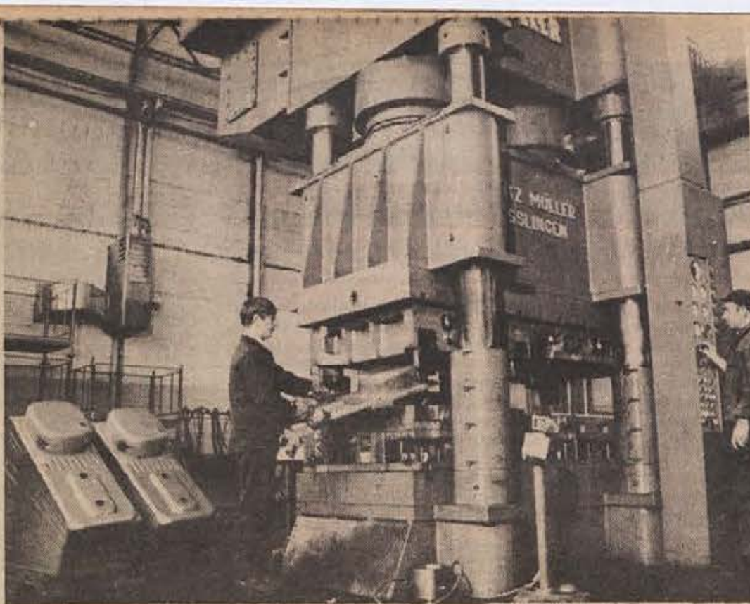
V okviru proizvodnje gospodinjstve opreme izdeluje Industrija motornih vozil tudi pomivalna korita nerjaveče pločevine. Izdelujejo enodelna in dvodelna korita z odcejalnikom. 14.000 jih bodo vgradili stanovanjske priklovice, ostalo proizvodnjo pa namenili široki potrošnji. (Foto: M. Vesel)
