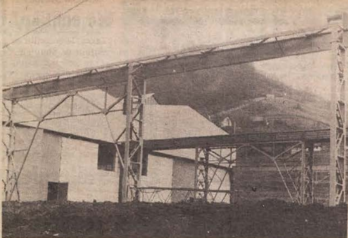
Še dober mesec in 4000 kvad. metrov velika tovarna gradbenih žerjavov na Senovem bo začela obratovati. Trenutno napeljujejo v njej električne priključke, nakar bodo začeli polagati pode. Prijave za namestitve v novem obratu Metalne že prihajajo. Prednost bodo seveda imeli bivši rudarji. (Foto: Jožica Teppey)
