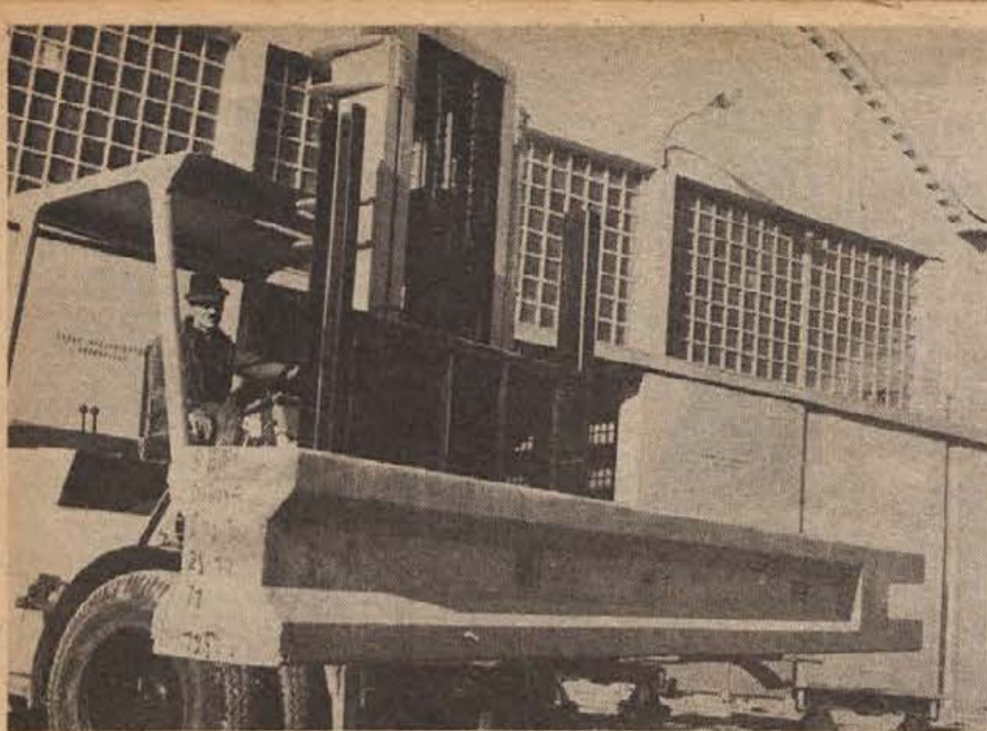
Takle je železobetonski steber za bodočo Betino halo v Dobovi. Z velikim viličarjem prenašajo gotove izdelke. V ozadju se vidi tovarna Togrel v gramoznici pri Krškem.
