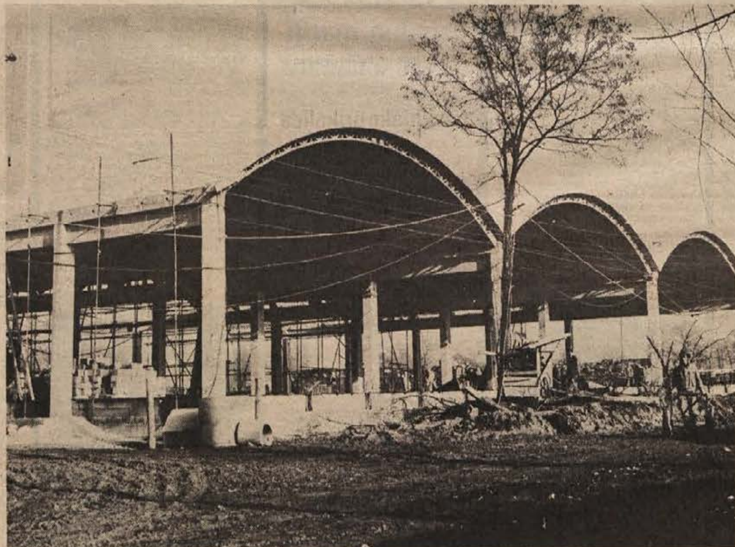
Pogled na sklop montažnih hal na Pionirjevem gradbišču v Zagrebu. Železobetonske elemente so izdelali v svoji tovarni v Krškem in jih zatem prepeljali na gradbišče. Prednosti: hitra gradnja in vsestranska uporabnost. (Foto: M. Vesel)
