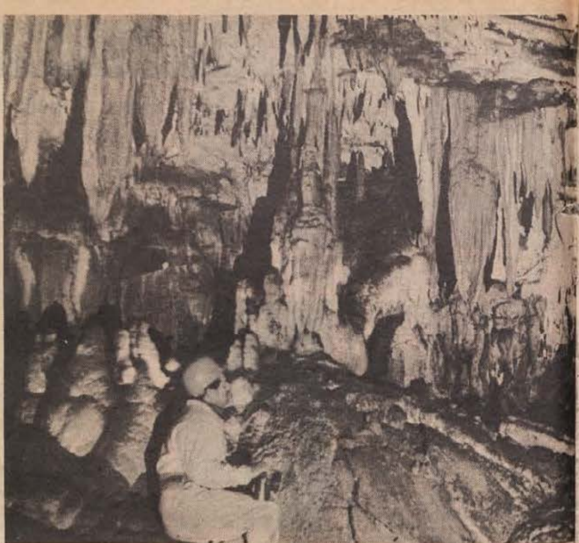
Tole kraško skupino v prvi dvorani so jamarji začasno krstili za „oltar“. (Foto: J. Primc)
