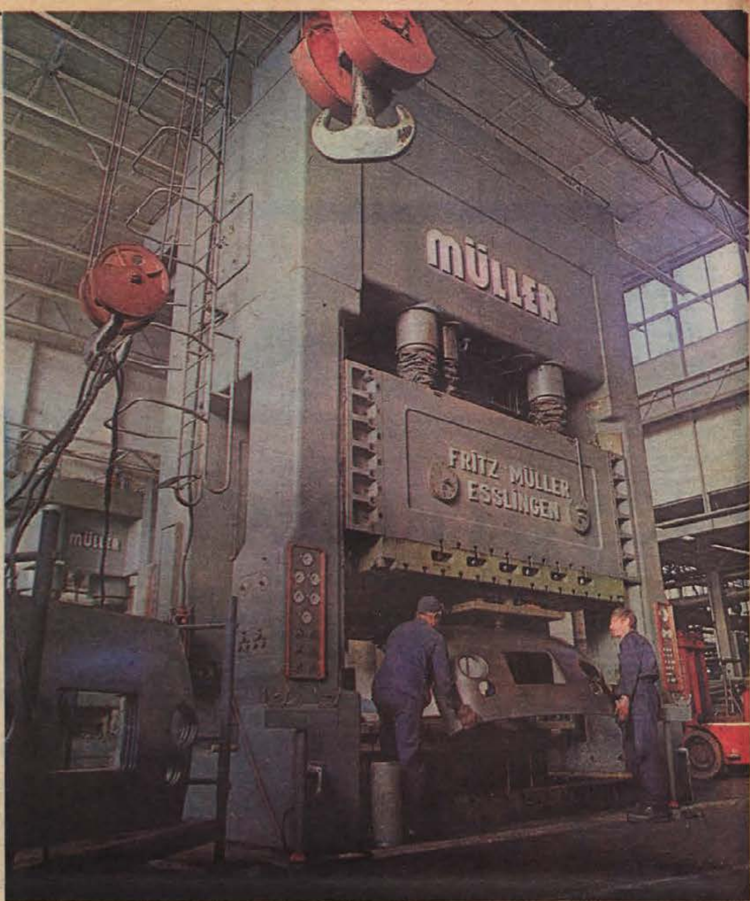
Orjaška preša s pritiskom 1000 ton oblikuje lahko vse karoserije iz proizvodnega programa IMV
