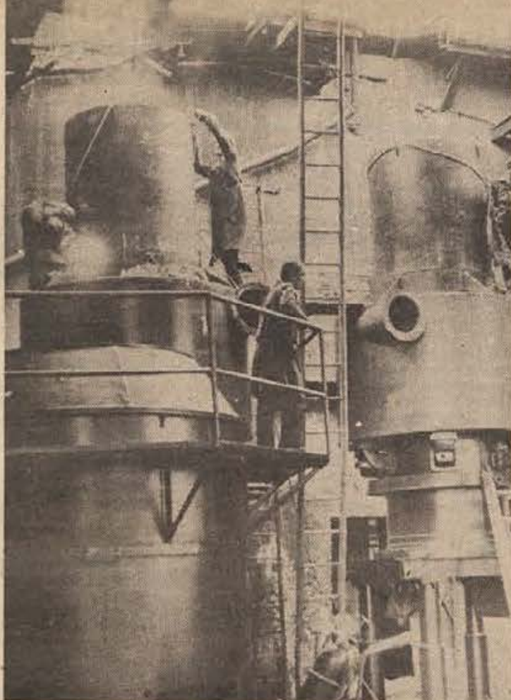
V črnomaljski tovarni COSMOS-BELT opravljajo montažo novih talilnih peči, ki so jih v celoti izdelali doma. Po sistemu cepljene litine bo omogočena proizvodnja mnogo boljše kakovosti, kar zagotavlja podjetju uspešen konkurenčni boj na tržišču. (Foto: R. Bačar)
