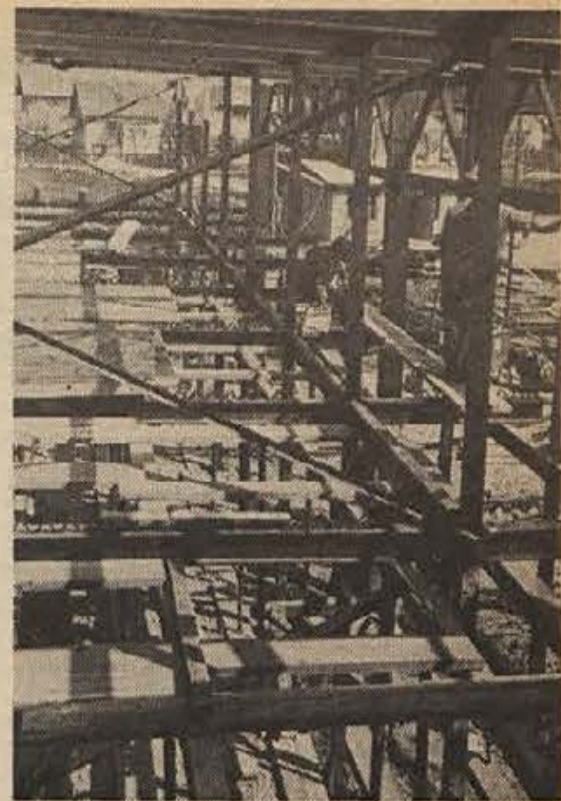
Tovarna pohištva v Brežicah bo konec junija dobila novo proizvodno halo, veliko 1.400 kvadratnih metrov. Z opremo vred bo veljala štiri milijone dinarjev. Železno konstrukcijo zanjo postavlja beograjsko podjetje, ker je dalo najcenejšo ponudbo (Foto: J. Teppey)
