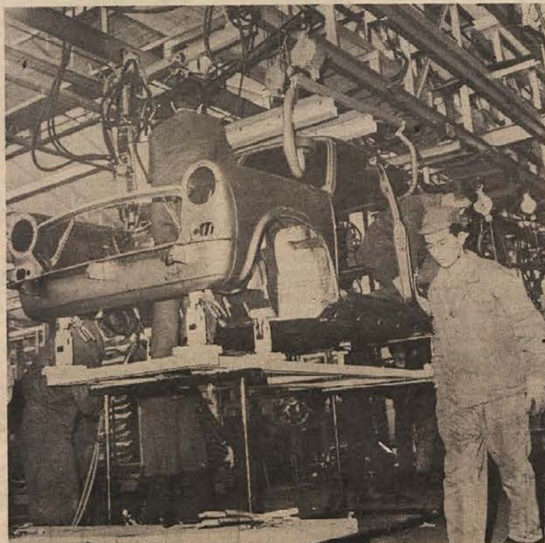
Tako nastaja na sodobnem tekočem traku pod elektrodami varilcev IMV 1300. (Foto: M. Moškon)
