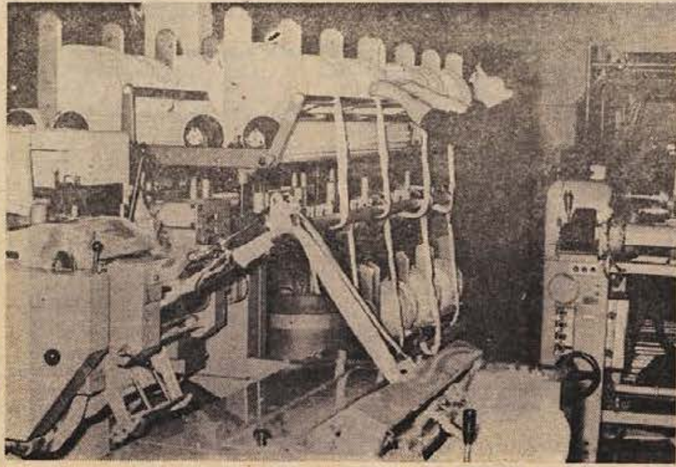
V metliški Novoteksovi predilnici imajo najsodobnejše predilne stroje. Raztezalka (na sliki), ki so jo uvozili iz Italije, sodi med zadnje dosežke v tekstilni industriji (Foto: S. Dokl)
