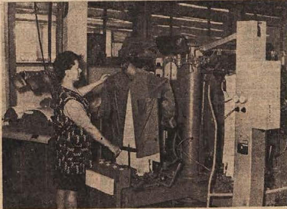
Tale likalni stroj, pravijo mu »permanentprese«, so dobili pri LABODU šele pred nedavnim. Brez zamudnega zlaganja in obračanja zlika srajco na mah na stoječem modelu, na katerega jo je pravkar naravnala delavka na levi strani slike
