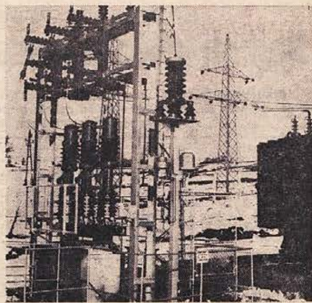
11. februarja ob 13. uri je začela obratovati novo-zgrajena razdelilna transformatorska postaja v Črnomlju, s pomočjo katere bo odpadla marsikatera pripomba na račun slabega električnega toka v Beli krajini. Podjetje Elektro je investiralo v gradnjo in daljnovod okoli 318 milijonov Sdin, gradilo je domače gradbeno podjetje BEGRAD, opremo pa je dobavila Hidromontaza iz Maribora.
