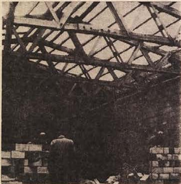
Predvideno je, da bo do prvega maja prihodnjega leta dokončana rekonstrukcija sevniške Kopitarne. Tovarna bo dobila nove prostore za izdelavo kopit in obrat za izdelavo pet ter še nekatere druge prostore. Kolikšno je gradbišče, pove podatek, da izvajalec del gradbeno podjetje iz Zagorja gradi in obnavlja na okoli 3500 m 2 zidanih površin. Na sliki je del novega obrata za izdelavo kopit. (Foto: M. Legan)
