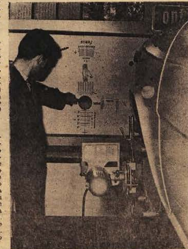
Kontrola stežkanja koles (špura) na optični napravi, na kateri se kontrolira tudi celotno podvožje osebnega avtomobila. (Foto: Mirko Vesel)
