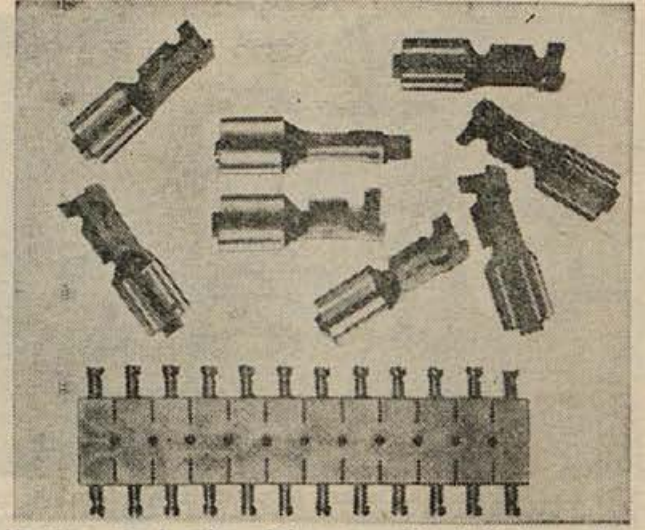
Na dnu gornje slike vidite posamične kabske spojke, kakršne dela novomeška ELA, na vrhu slike pa so te spojke v 12-polni spojni letvi
