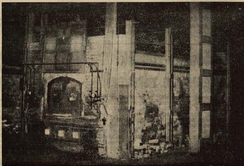
Ce si boste ogledali gornjo sliko, si boste laže predstavljali, kaj je to temper peč. Na sliki je namreč ena izmed obeh temper peči, ki sta povzročili toliko škode v novomeški INIS. V tej peči segrejejo šobe na 1500 stopinj C, nato jih pustijo v njih, da se ohladijo na 900 stopinj C, ter prenesejo nekaj metrov daleč v kadno peč, kjer jih spustijo v razbeljeno tekoče steklo. Šobe se zaradi svoje specifične teže ne potopijo v steklo, pač pa plavajo po njem, skozi podolžno odprtino v šobah pa nato vlečejo z vlečnimi stroji steklo kvišku. (Foto: Miloš Jakopec)
