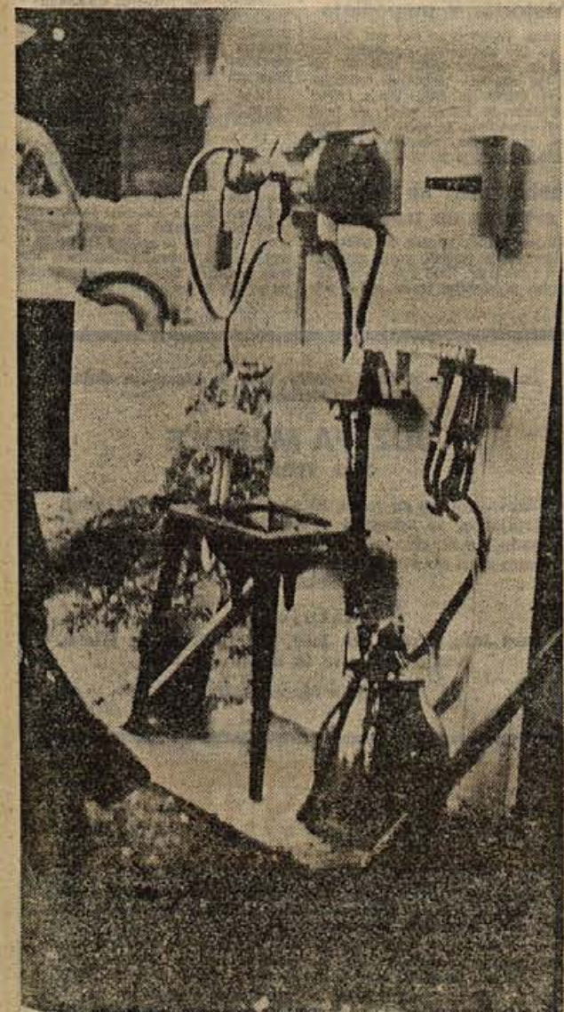
MOLZNI STROJ — Kateri rejec krav ne bi želel imeti v hlevu molznega stroja? Pri nas jih v zasebnih hlevih še ni, čeprav je molza zelo naporno kmečko delo. Na sliki je prenosna molzna naprava, izdelek vodeče tvrdke Alfa Laval, ki je namenjena številu krav (4—12). V manjših kmetijskih obratih je pri severnih sosedih že zelo razširjena. (Foto: M. Legan)
