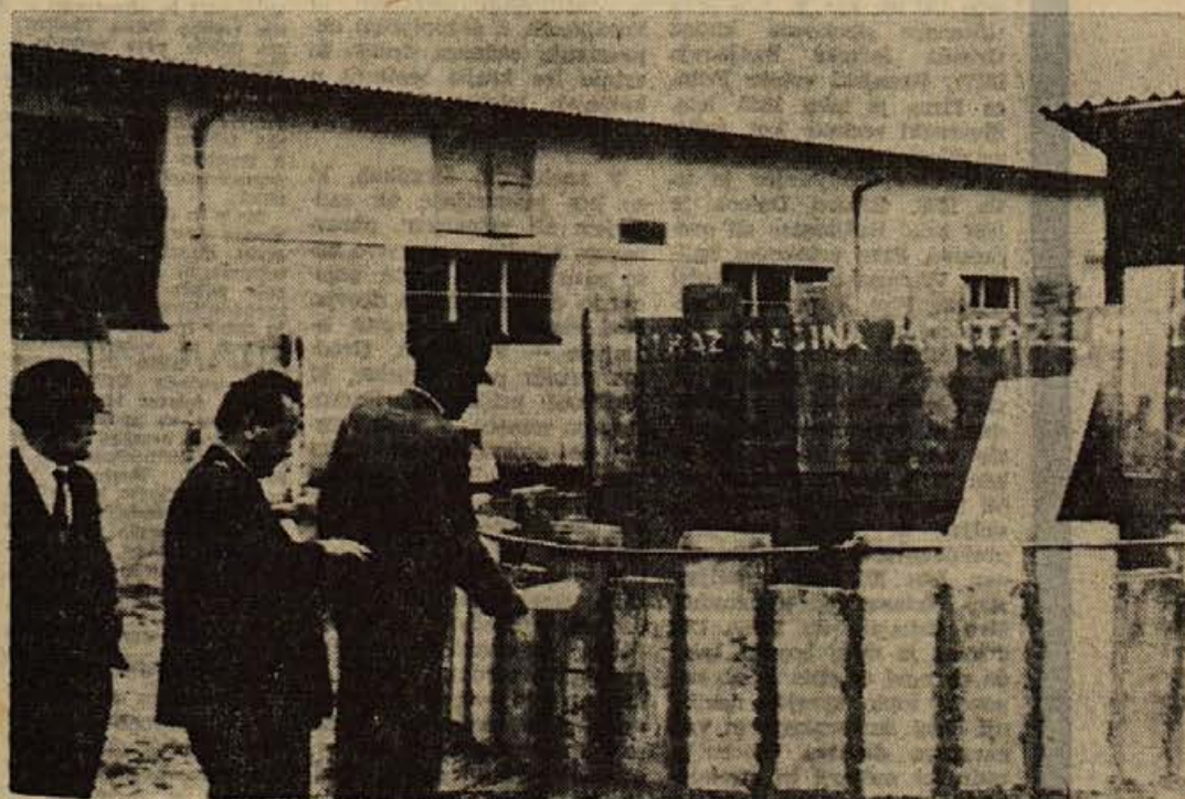
Ce bi imel primeren kalup, bi si lahko vsak kmetovalec sam naredil montažni silos, kakršne prodaja gradbeno podjetje Dravograd. Njegov silos, ki ga prikazuje gornja slika, ima premer 3 m in višino 6 m, vanj pa gre 45 m 3 silaže. Pokrit je z leseno streho.
