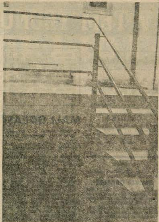
To je ograja na stopnišču na Ljubljanski cesti 33 (in 31 ter 29) v Kočevju, skozi katero je padel 3-letni otrok. Ograja je visoka okoli 85 do 86 cm, razmaki med zgornjo, srednjo in spodnjo kovinsko cevjo znašajo kar 26, 27 in 23 cm! Je to »varnostna ograja« ali samo »ograjac«?
