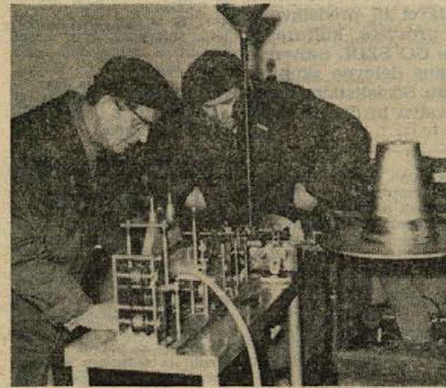
Konstruktor Tone Petrič (na levi) in mehanik Tone Suštaršič izdelujeta v ISKRINEM obratu uporov v Šentjerneju stroj avtomat za spajkanje uporov. Tudi ta novi avtomat bo veliko pripomogel k izdelavi velikih serij in izdelke pocenil (Foto: Miloš Jakopec)
