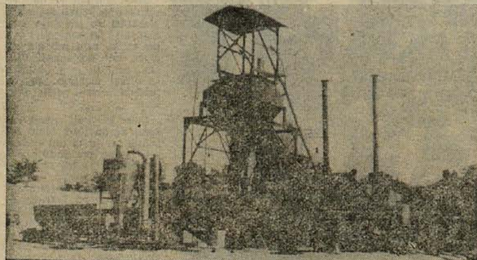
V gramoznici, pri odcepu avtomobilske ceste pri Krškem, je začelo Cestno podjetje iz Novega mesta letos graditi svojo asfaltno bazo. Tamkajšnji gramoz je zelo primeren za izdelavo asfalta, kraj pa je pri roki tudi za prevoze asfaltno mešanice na razna delovišča. V dveh pečeh lahko pripravijo od 32 do 36 ton asfaltno mase na dan, eno izmed obeh peči pa kanijo prodati.
